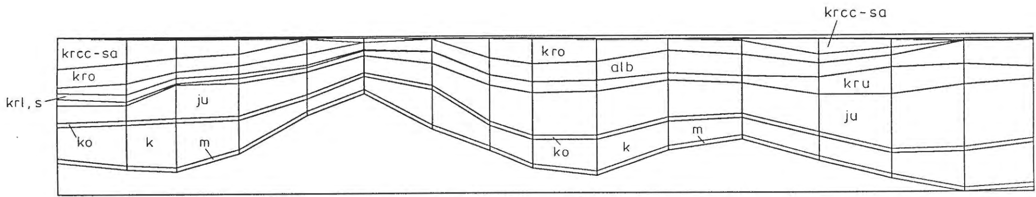
BILD 22: GEOL. PROFIL 7 – CFEST-GEOMETRIE
